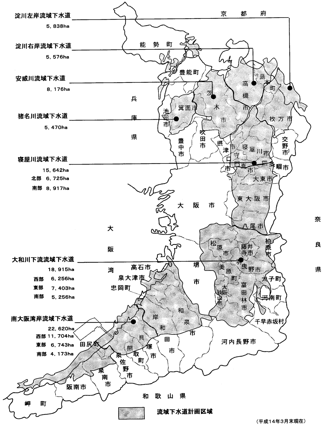
7-19 大阪府下水道計画概念図
