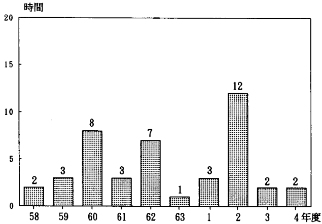
図 2-5-11 昼間の光化学オキシダント濃度が0.12ppm以上の時間数の平均の推移 (10年間継続局)
