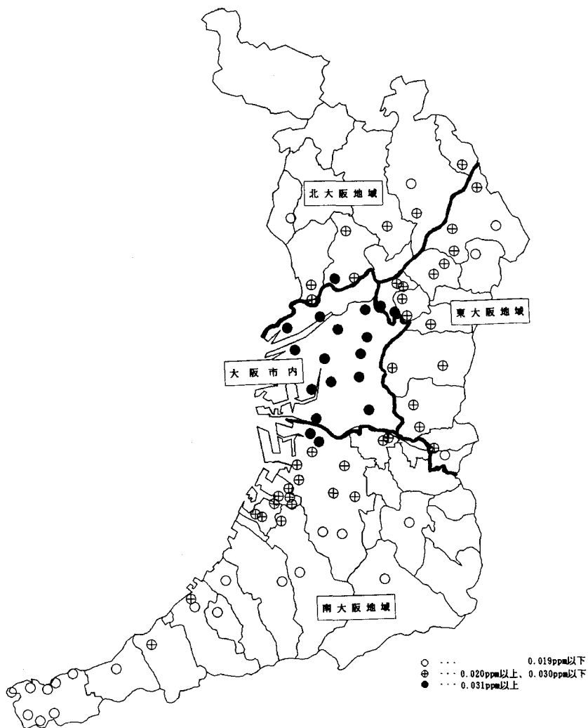
図2-5-1 一般環境測定局の二酸化窒素濃度（年平均値）の概要（平成4年度）
