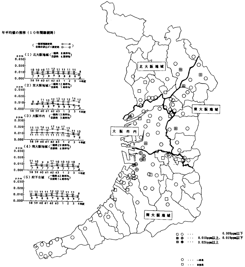
図 2-5-17 二酸化硫黄濃度（年平均値）の概要（平成4年度）と推移
