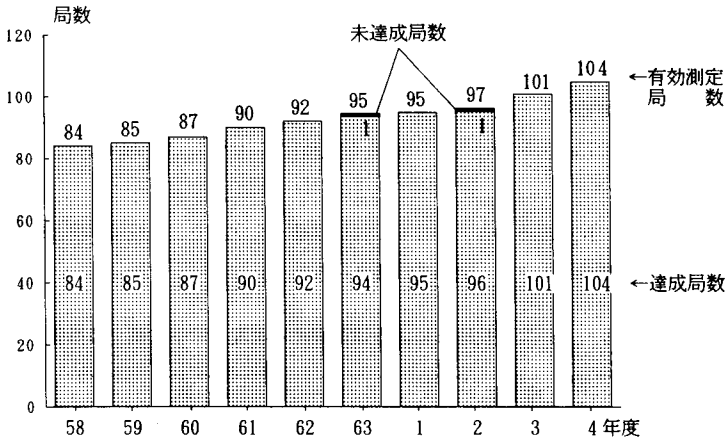
図2-5-18 二酸化硫黄の環境基準達成状況（長期的評価）の推移
