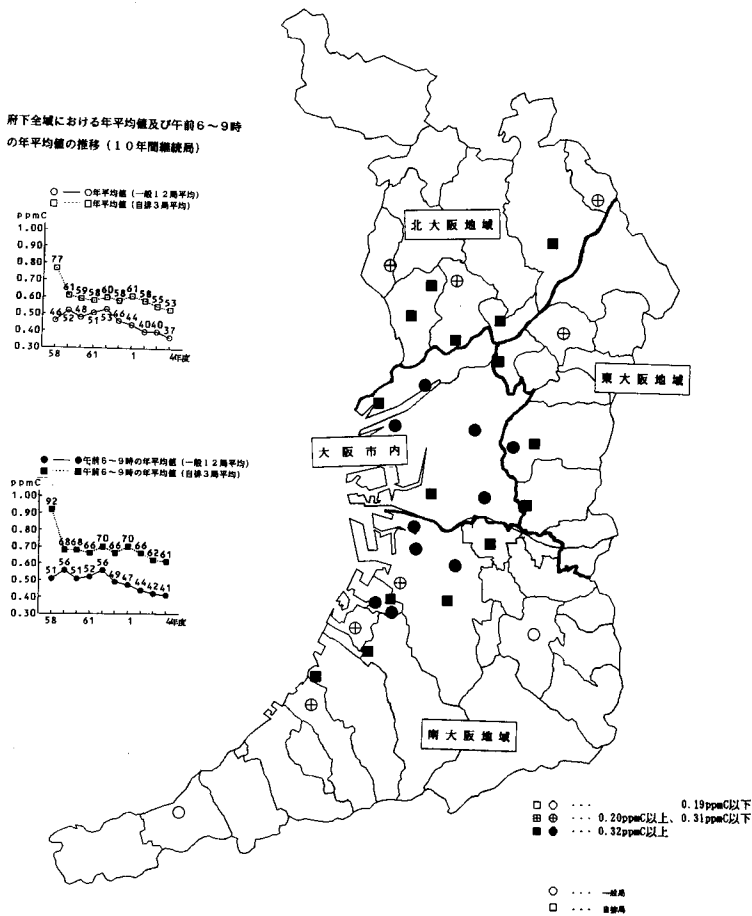
図2-5-14 非メタン炭化水素濃度（年平均値）の概要（平成4年度） と推移（年平均値及び午前6時から午前9時の年平均値）
