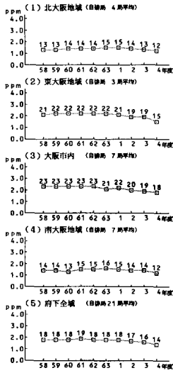
自動車排出ガス測定局の年平均値の推移 （10年間総観局）
