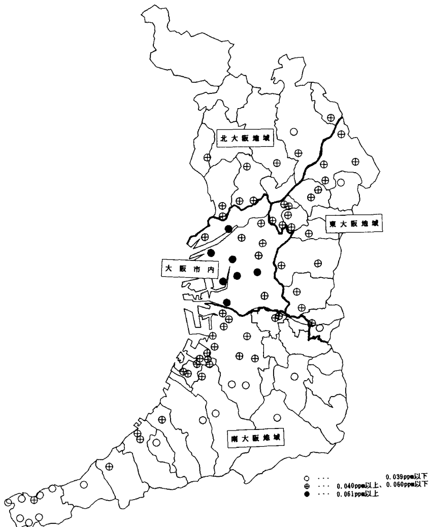
図2-5-4 一般環境測定局の二酸化窒素濃度（日平均値の年間98％値） の概要（平成4年度）
