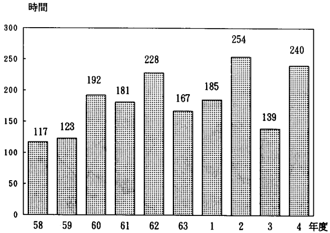
図 2-5-10 昼間の光化学オキシダント濃度が0.06ppm を超えた時間数の平均の推移 (10年間継続局)
