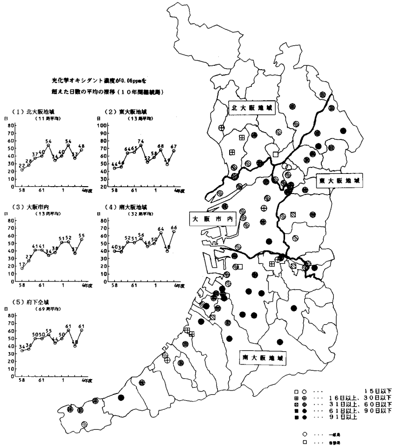
図 2-5-9 光化学オキシダント濃度（昼間1時間値）が0.06ppm を超えた日数の概要（平成4年度）と推移
