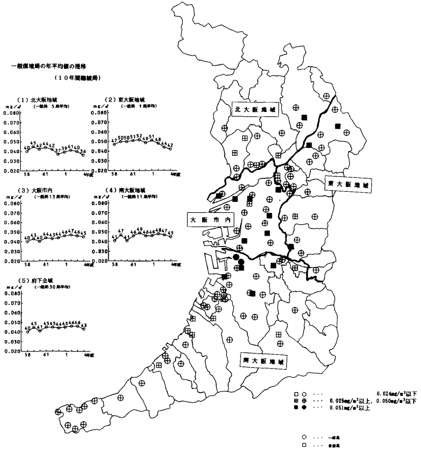
図2-5-15 浮遊粒子状物質濃度(年平均値)の概要(平成4年度)と推移
