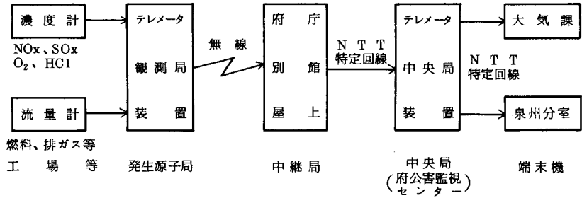
図 2 - 2 - 2 0 大気汚染発生源常時監視システムの概要
