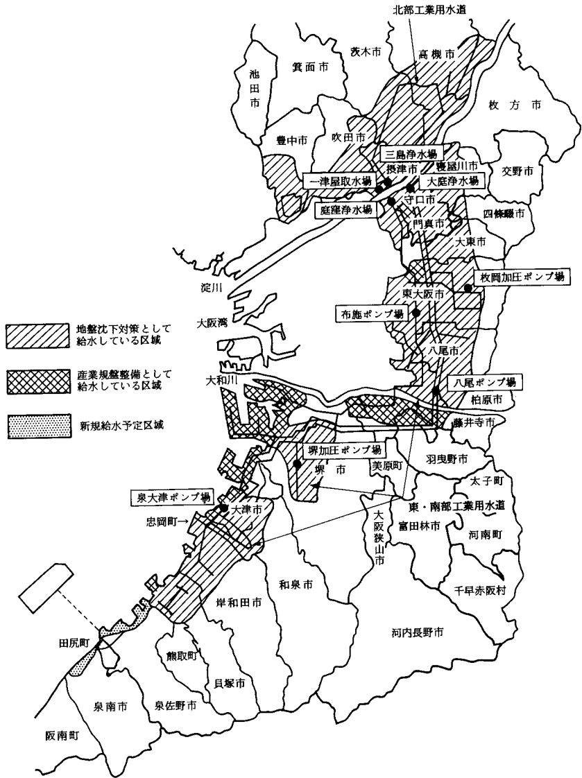
図2-7-7 府工業用水道が給水している区域
