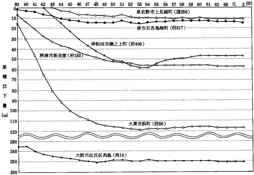
図 2-7-1 地盤沈下の推移
