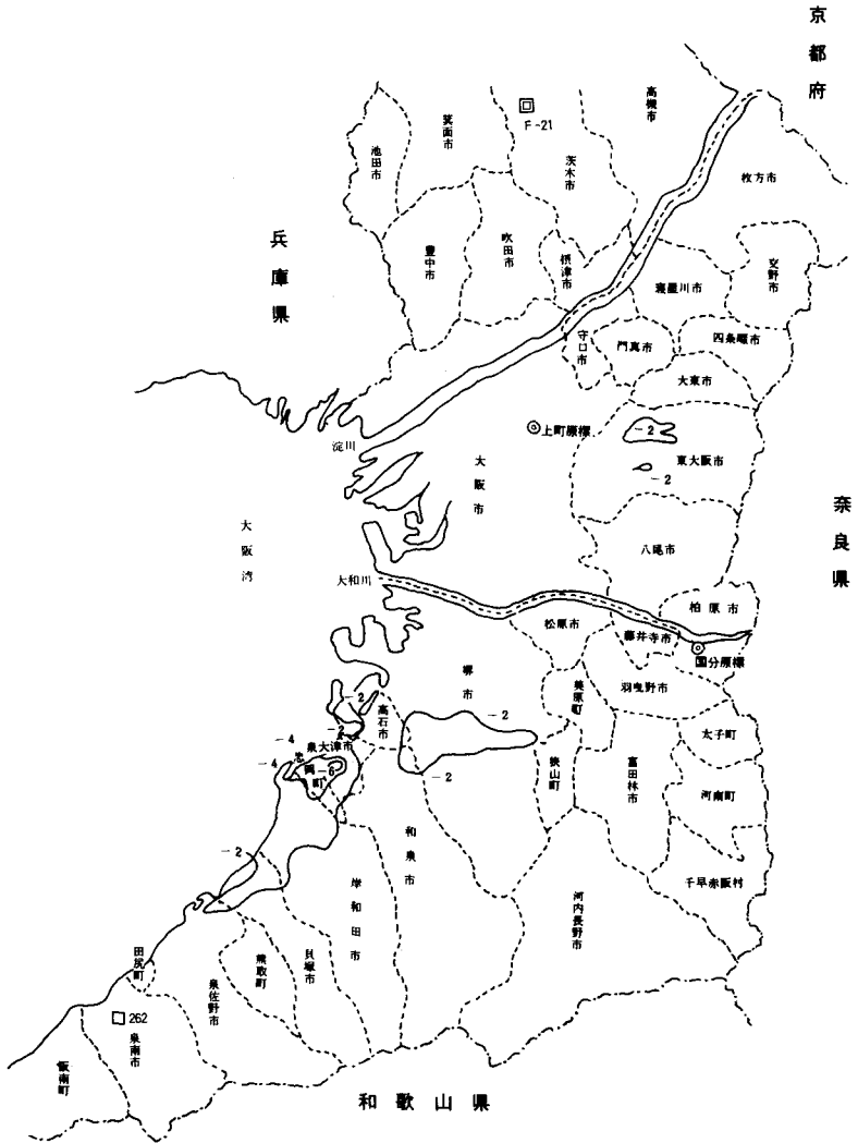
図2-4-1 地盤沈下等量線図
