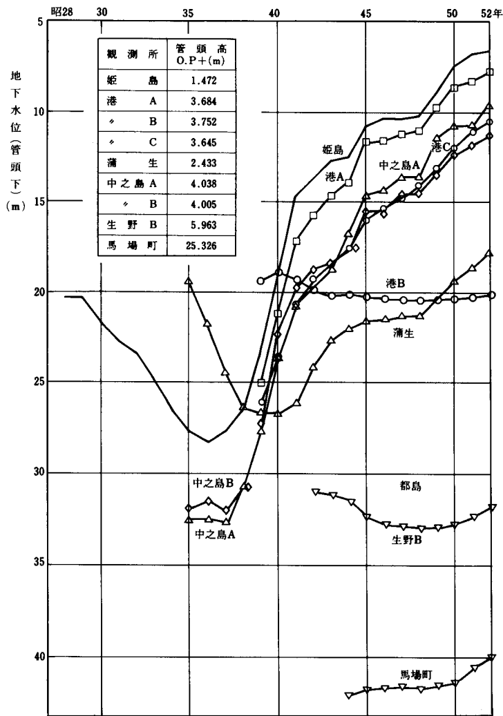
図2-4-3 地下水位の経年変化
