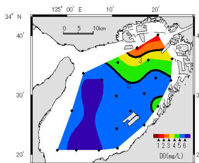
夏季底層 DO の分布図 (2017～2019 年度平均)
