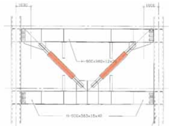
ダンパーの形状イメージ
