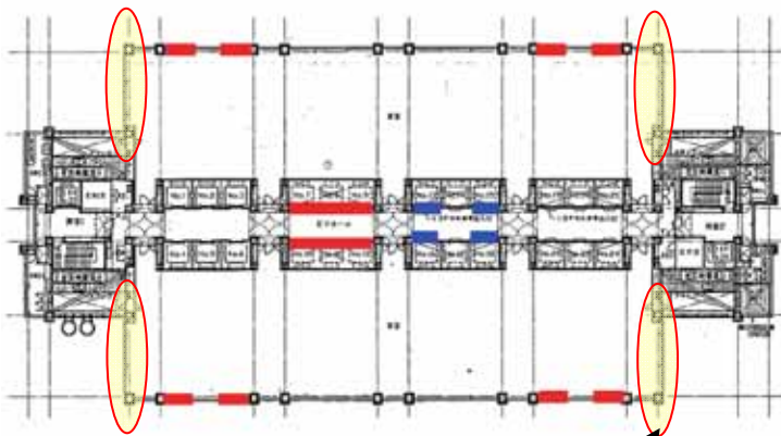
短辺方向ダンパー設置位置案
