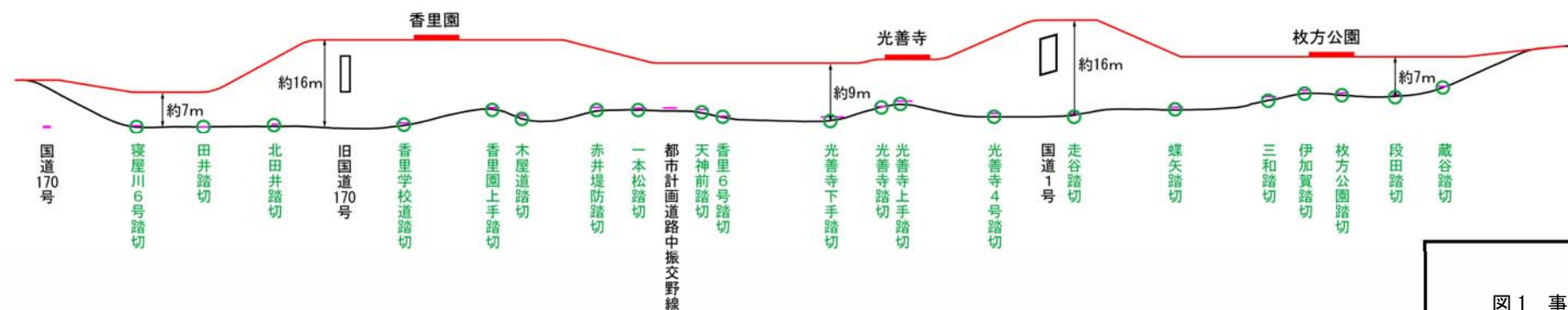
図1 事業計画（平面・縦断）
