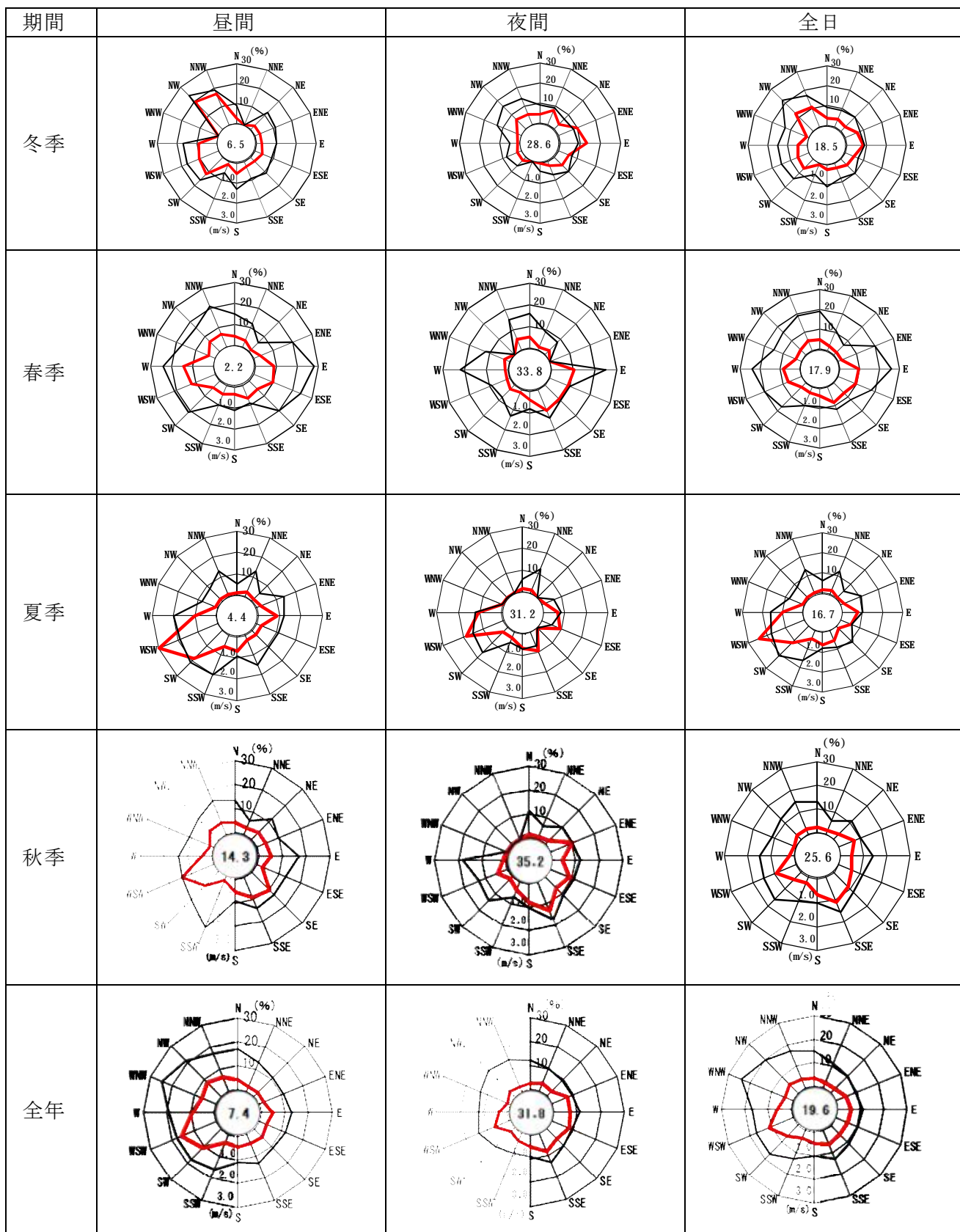
図4 風配図
