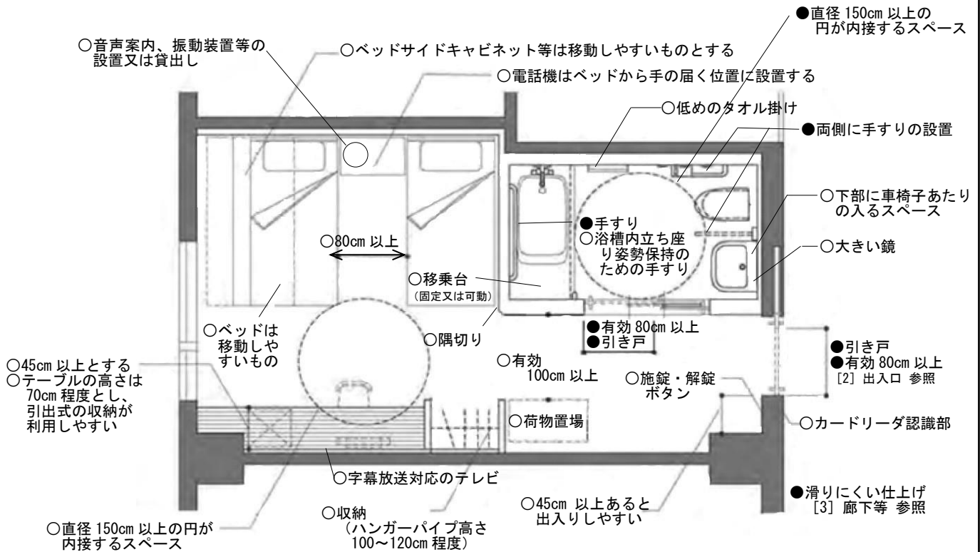
●○図 10.2 車椅子使用者用客室（ツインルーム）の例
