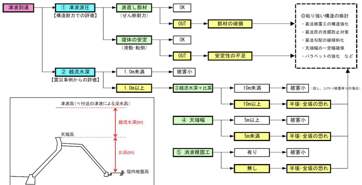
図 4-4 検討フロー（海岸）
