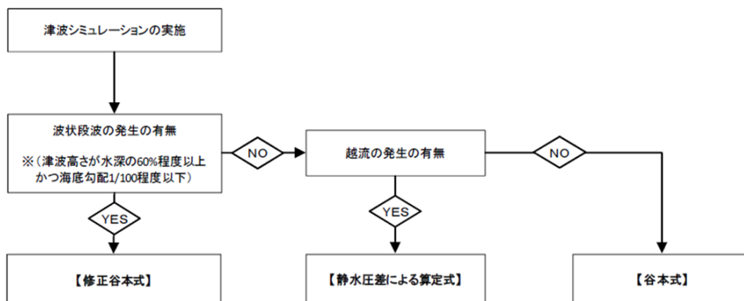
図3-22 津波算定式の選定フロー
