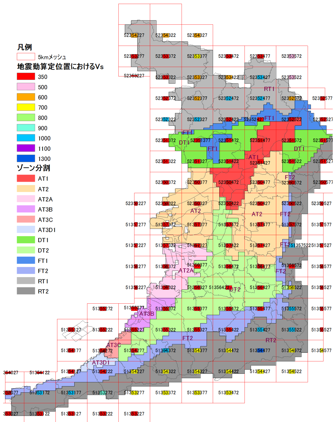
図2-2 メッシュ図
