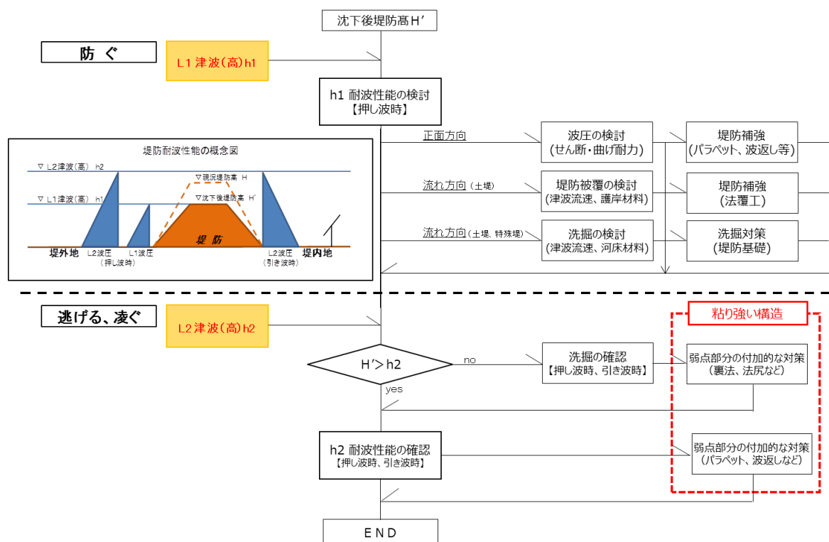
図2-12 検討フロー
