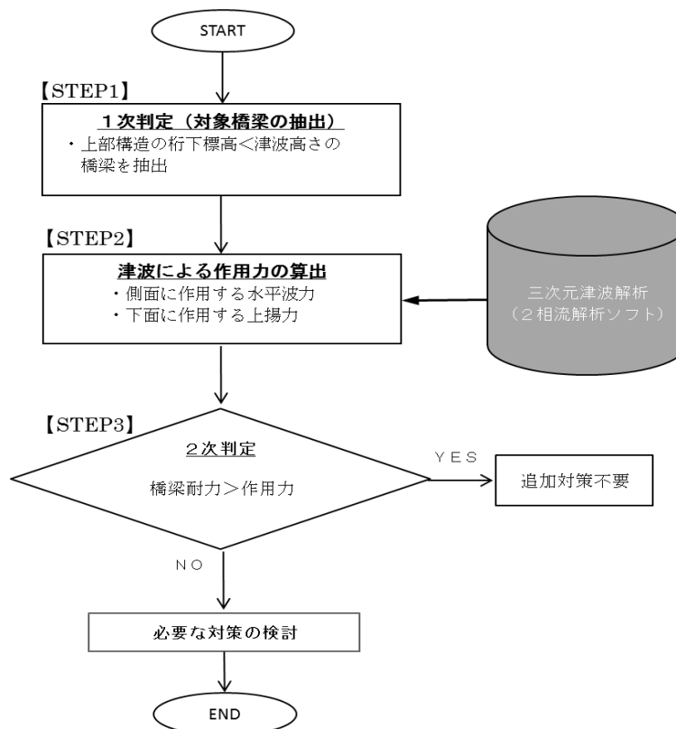
図2-14 点検フロー
