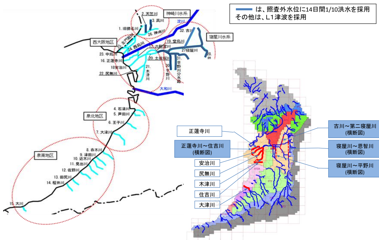
図 3-1 診断位置図（河川）
