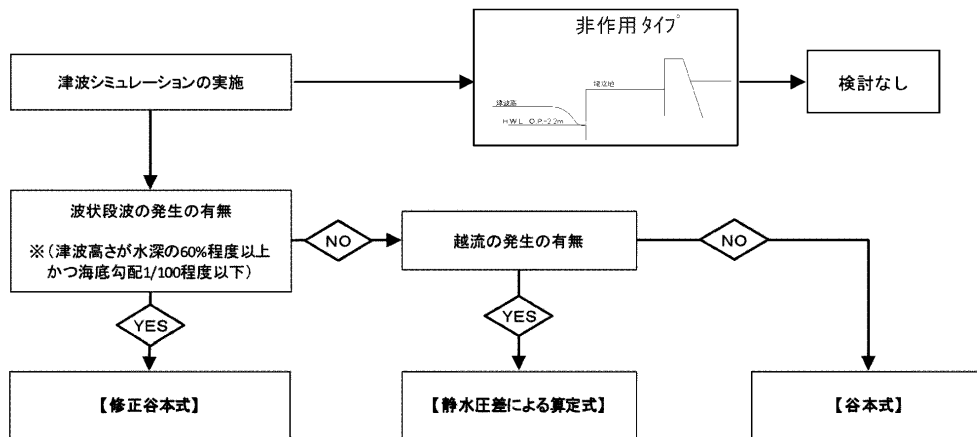
図3-23 津波波力算定の手順
