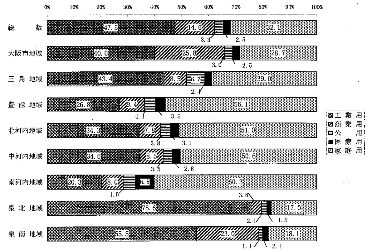
地域別都市ガス消費量の構成比 (平成10年度)
