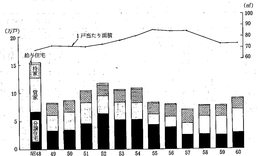
新設住宅数と1戸当たり延べ面積の推移
