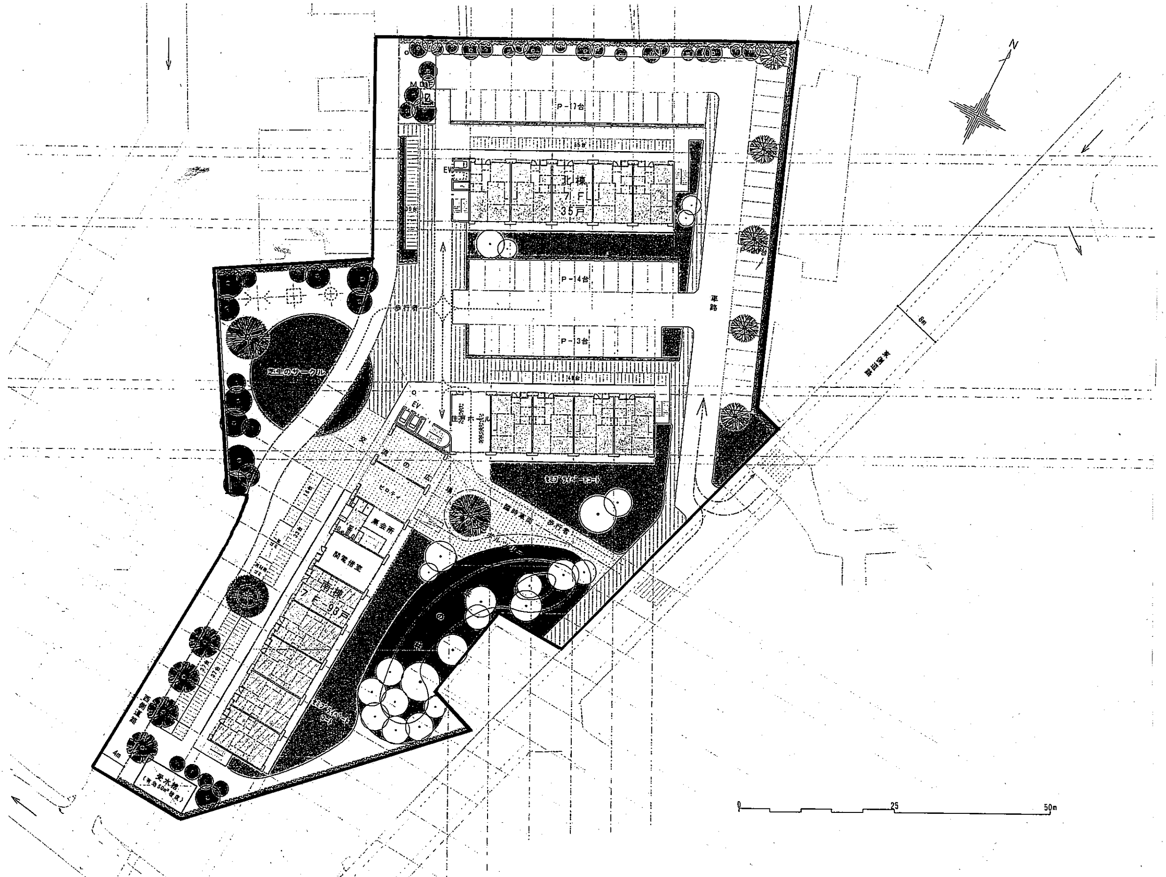
計画図
